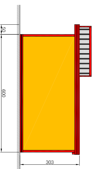
PROSPETTO LATERALE
