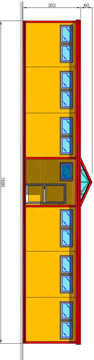
PROSPETTO PRINCIPALE
